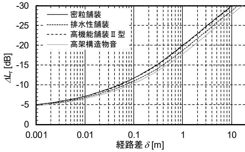
図-3.15 \Delta L_r と経路差 \delta の関係
